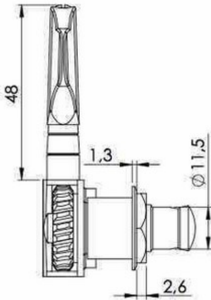
Seitenansicht von rechts side view right
