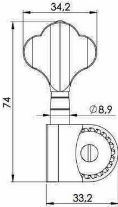
Vorderansicht front view
