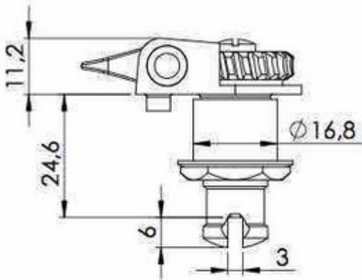
Seitenansicht von rechts side view right
