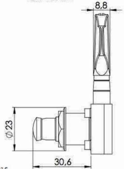
Seitenansicht von links side view left
