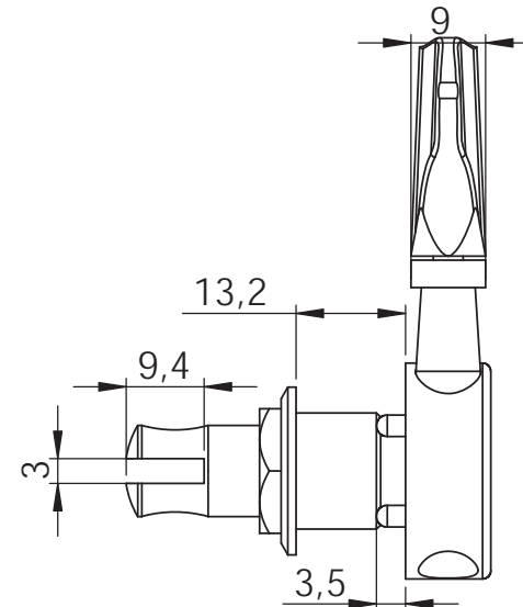
Seitenansicht von links side view left
